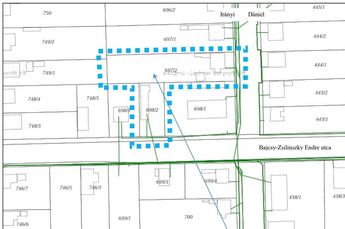
Gönyű, a Bajcsy-Zsilinszky Endre utcai hírközlési hálózat közművek/
